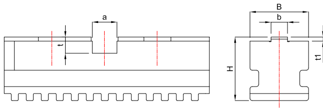
Grondbekken - specificaties
