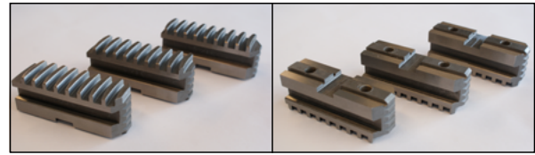
Grondbekken - specificaties
